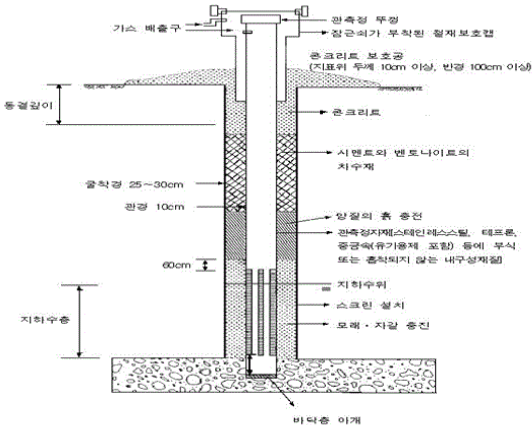
○ 조사항목 및 조사주기의 적정성 여부를 검토하여야 한다. - 조사항목 : 「지하수의 수질보전 등에 관한 규칙」 [별표4]의 생활용수수질기준 항목 - 조사주기 : 「지하수의 수질보전 등에 관한 규칙」 제6조제1항에 매립시설 사용종료 후 3년까지는 월 1회 이상 조사 - 지하수 오염관측정 설치방법 : 「지하수의 수질보전 등에 관한 규칙」 제3조제2항 [별표3] 지하수오염관측정의 설치방법 및 지하수 오염관측정의 구조도에 따라 설치 6) 주변해역 수질조사계획(해수면 인접매립시설에 한함) ○ 매립시설 인접해역의 수질조사항목 및 조사주기 등의 적정성 여부를 검토하여야 한다. - 조사항목 : 「환경정책기본법」 시행령 [별표] 해역환경기준 - 조사주기 : 분기마다 1회 이상 조사 여부 - 조사지점 : 매립시설을 접한 해안선을 따라 육지 끝으로부터 일정거리별로 최소 2개 이상의 조사지점 선정 여부
